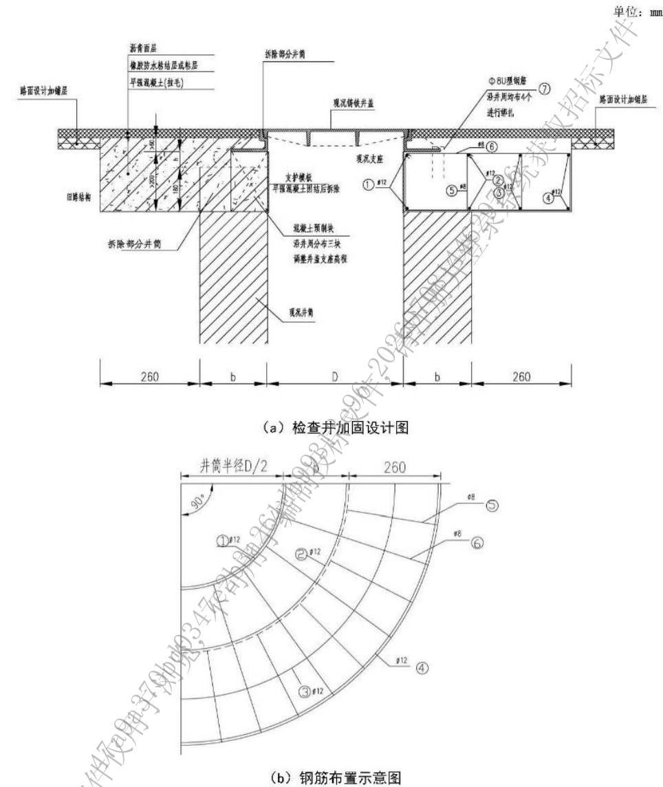
图1 检查井加固构造图（钢筋混凝土加固）
