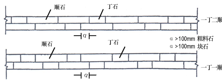
镶面石砌筑
