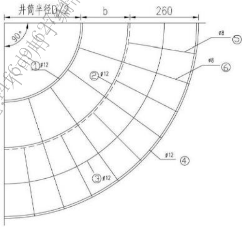
(b) 钢筋布置示意图
