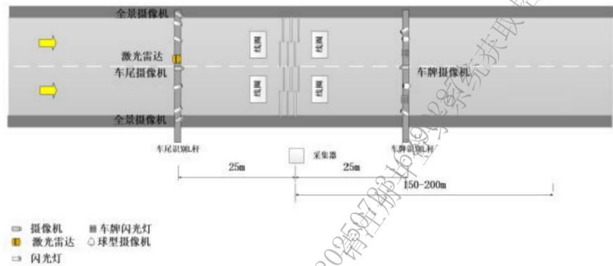
图 A.1 公路货运车辆不停车超限检测系统典型布局
