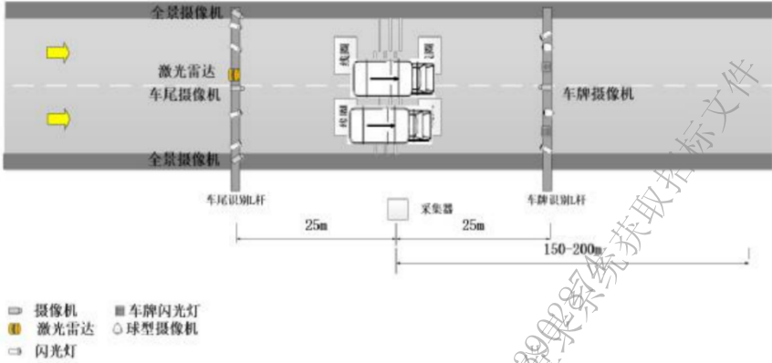
图 B.3 双车并行（一车跨道）
