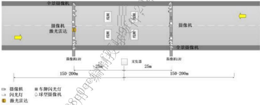
图 C.4 双向 2 车道
