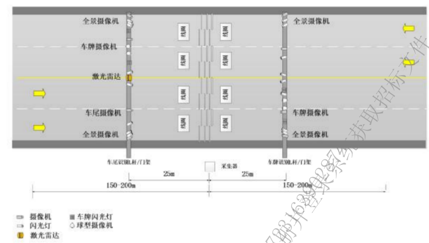
图 C.5 双向4车道
