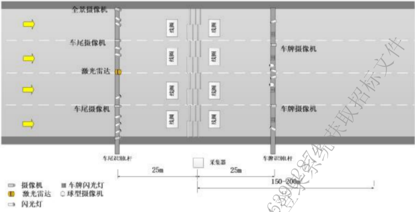
图 C.3 单向 4 车道
