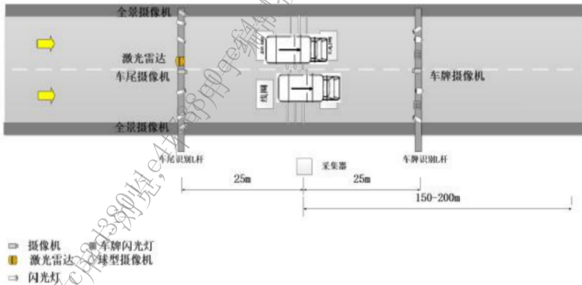
图 B.2 双车紧邻并行
