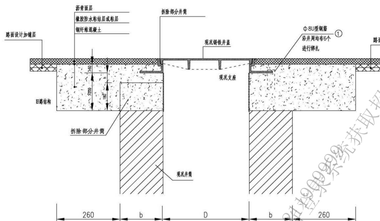
(a) 检查井加固设计图
