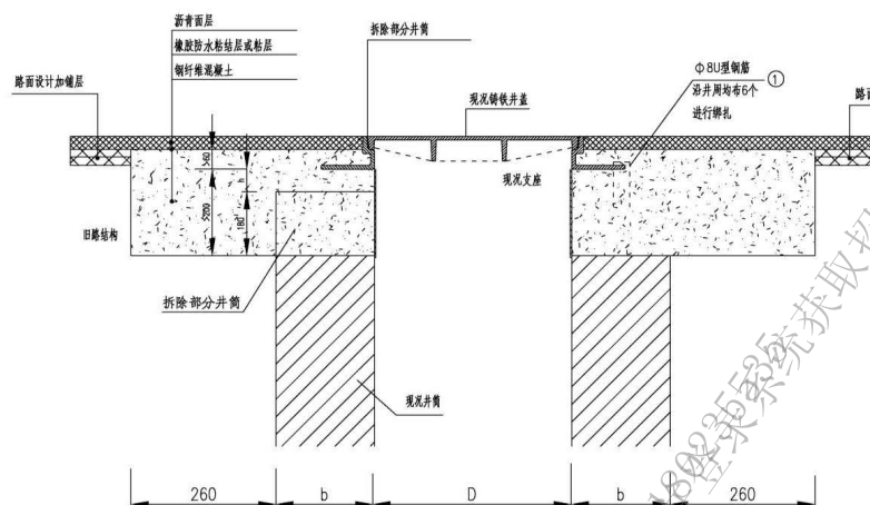
(a) 检查井加固设计图
