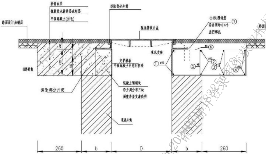
(a) 检查井加固设计图
