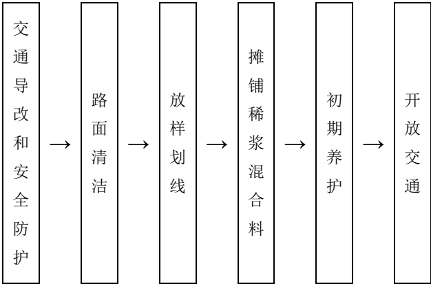
图18 稀浆封层和微表处施工作业的工艺流程
