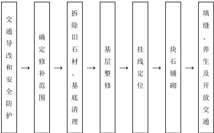
图10 块石路面维修的工艺流程
