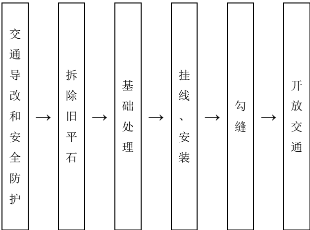
图16 平石维修作业的工艺流程
