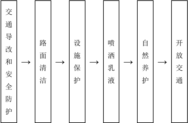
图19 雾封层施工作业的工艺流程
