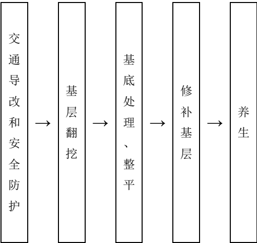
图14 基层维修工艺流程
