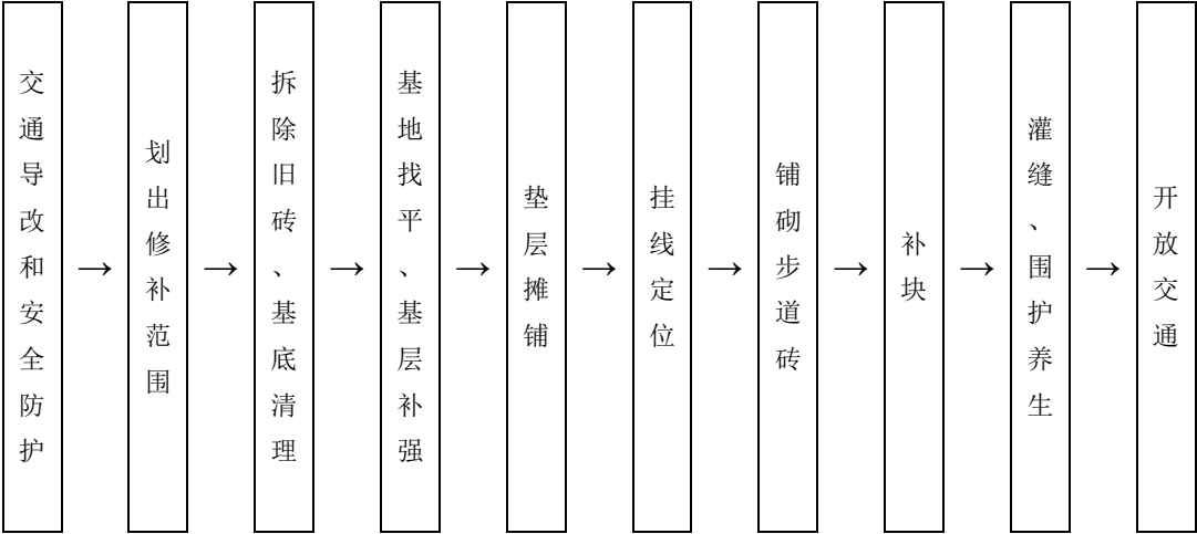
图12 普通水泥混凝土步道砖维修工艺流程
