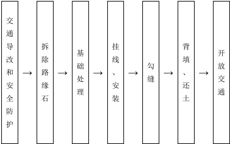
图15 路缘石维修作业的工艺流程
