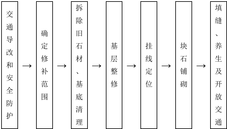
图11 砌块路面维修的工艺流程
