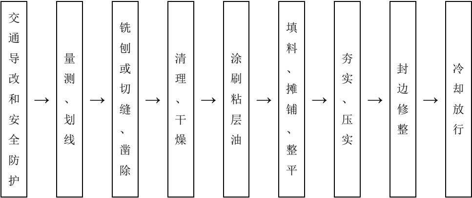
图4 坑槽热料修补的工艺流程
