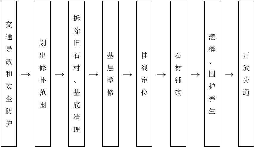
图13 石材步道砖维修工艺流程
