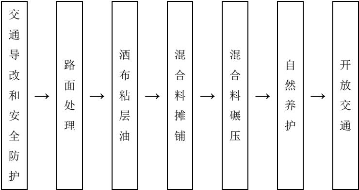
图17 薄层热拌沥青混凝土罩面施工作业的工艺流程
