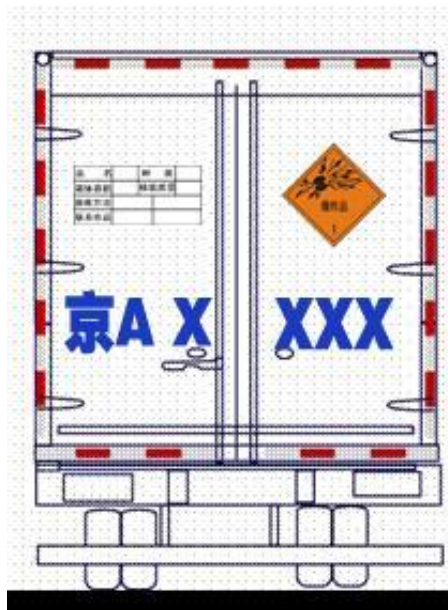
图 B.4 安全告示牌在厢式货车上的位置
