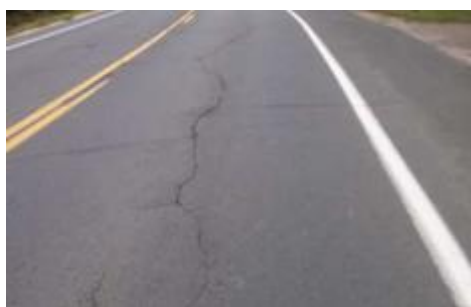
b) 轻度纵向裂缝
