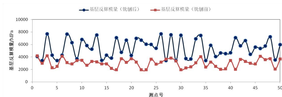
图 C.1 试验路半刚性基层模量对比
