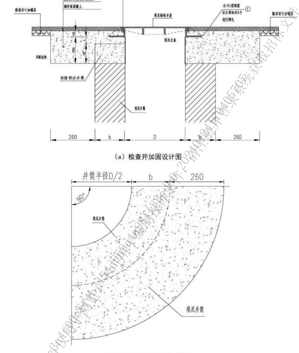
(b) 钢纤维混凝土布置示意图
