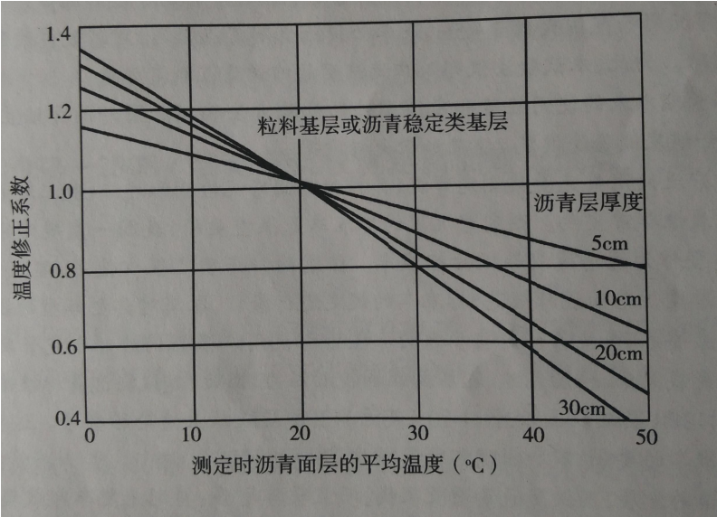
图 T 0951-3 路面弯沉温度修正系数曲线(适用于粒料基层及沥青稳定基层)
