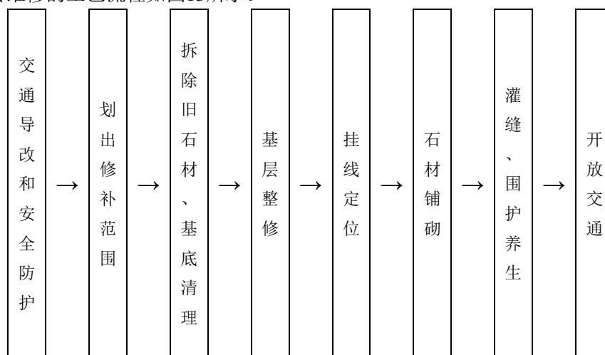
图13 石材步道砖维修工艺流程
