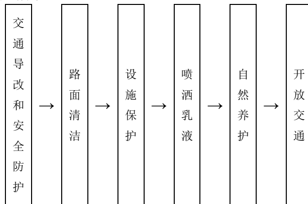
图19 雾封层施工作业的工艺流程
