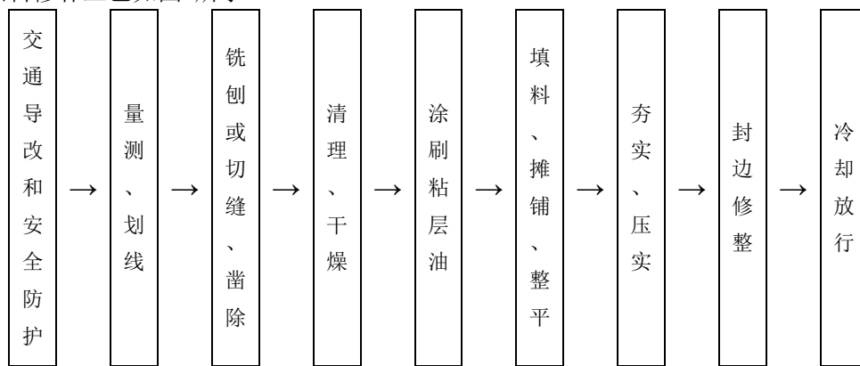
图4 坑槽热料修补的工艺流程
