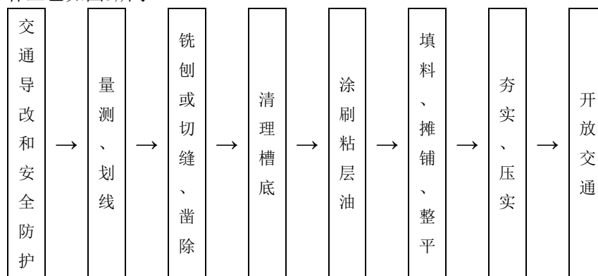
图5 坑槽冷料修补的工艺流程
