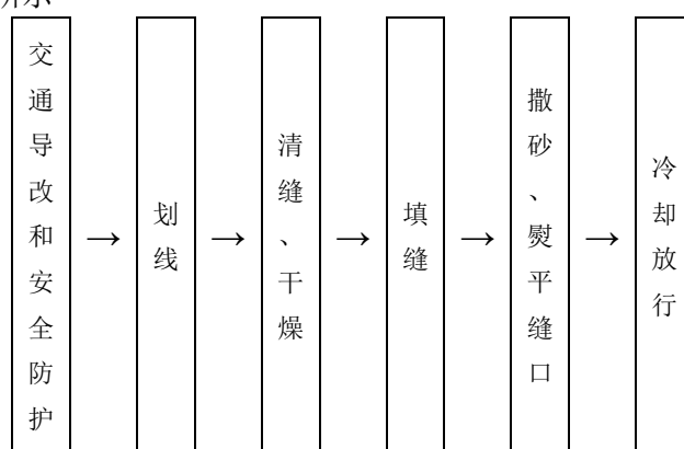
图3 沥青混合料填缝的工艺流程
