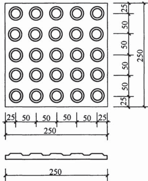
图 3-4 提示盲道
