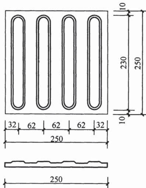
图 3-3 行进盲道
